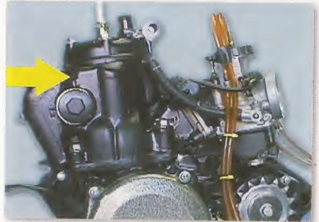
Motor de dos tiempos con refrigeración líquida
